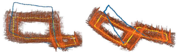
Fig. 8. Misaligned LiDAR SLAM.
