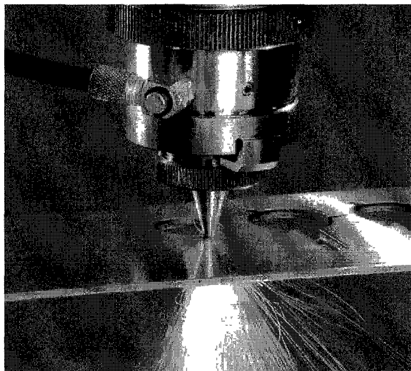
Snijden van CrNi band zonder oxidatie
