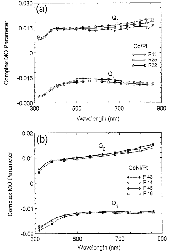
Fig. 5. Dispersion of the complex magneto-optic Voigt parameter \hat{Q} (= Q_1 + iQ_2) .
