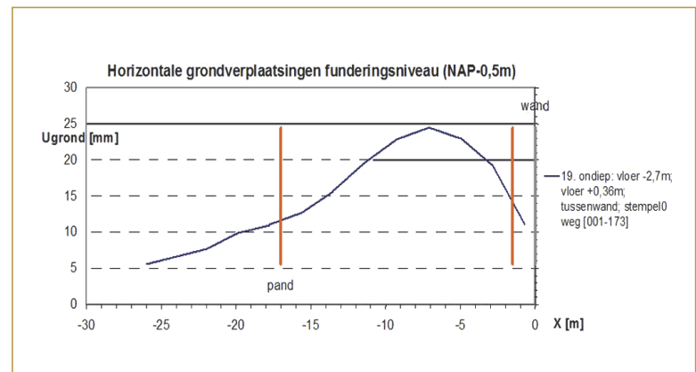
Figuur 8 – Horizontale grondverplaatsing op maaiveldniveau dsn c-c na maatgevende bouwfase.
