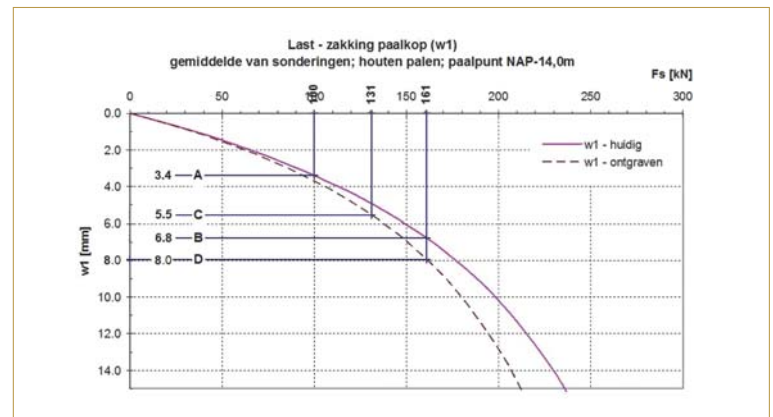
Figuur 12 – Last-zakkingcurve paalkop houten paal voor gemiddelde van de sonderingen.
